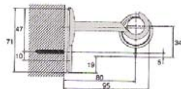
Support mural simple 80 mm avec base support allongé
