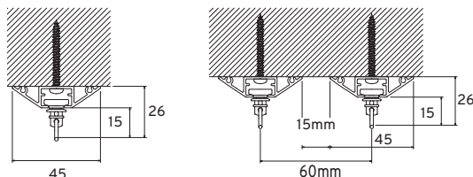
Fixation plafond directe simple et double
