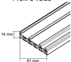
Profil 5 voies
